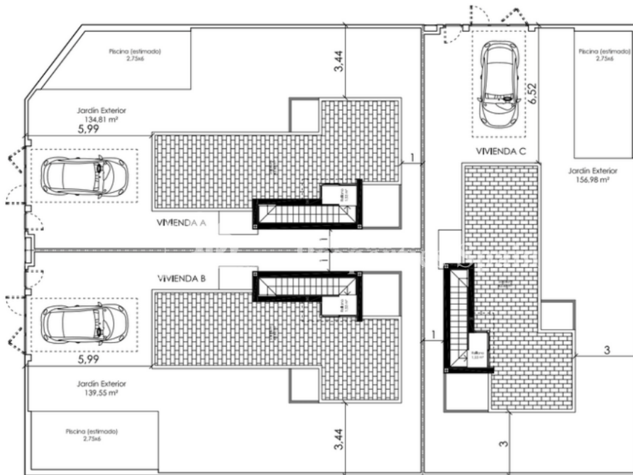
Planta Solarium
