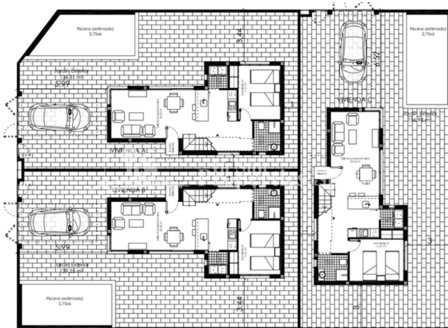
Planta Baja
