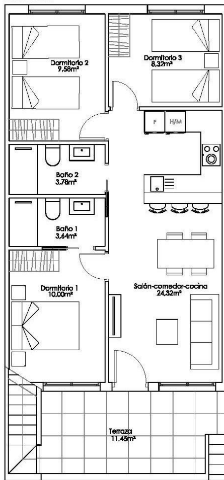
Planta Vivienda
