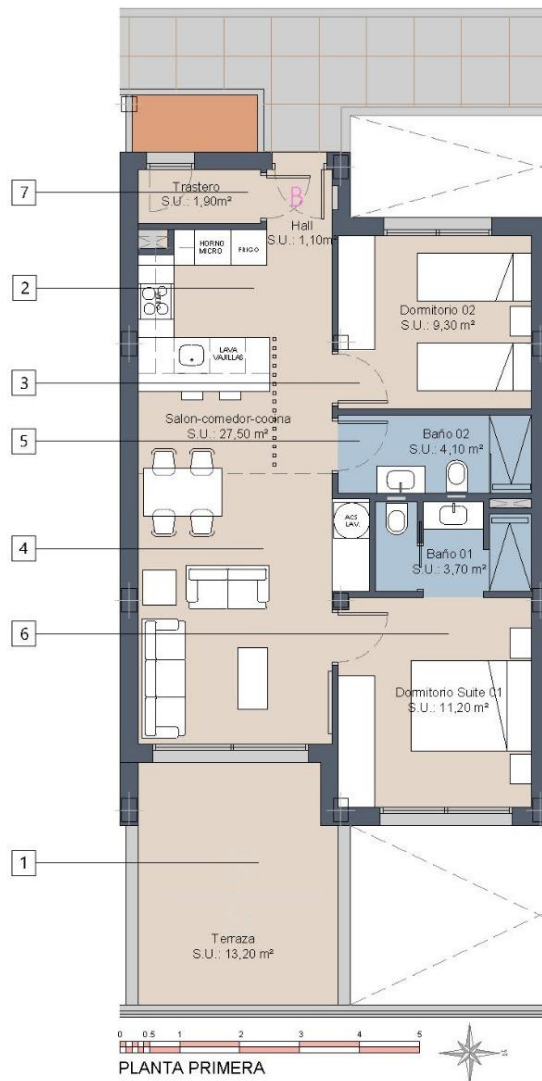
PLANTA PRIMERA
