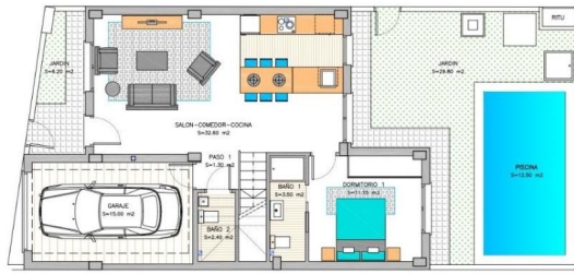
Planta Baja
