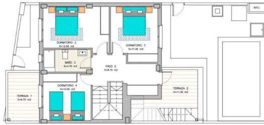
Planta Primera
