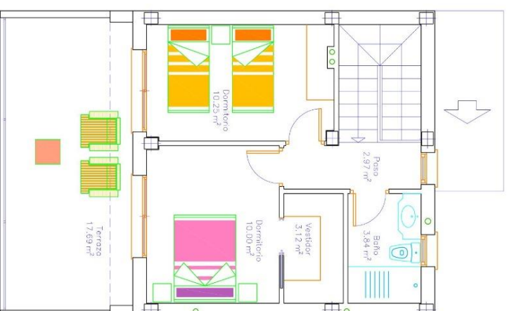
PLANTA 1
