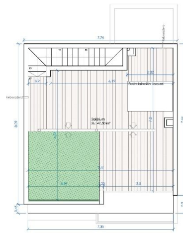
PLANTA CUBIERTA
