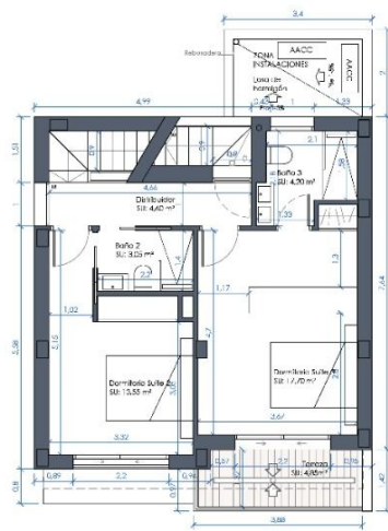
PLANTA PRIMERA
