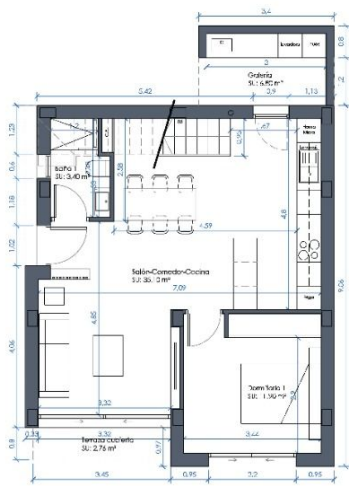
PLANTA BAJA
